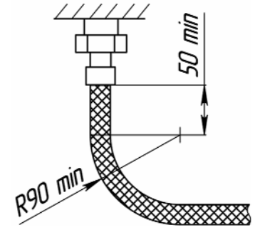
Рисунок 7. Требования к изгибам гибких шлангов
