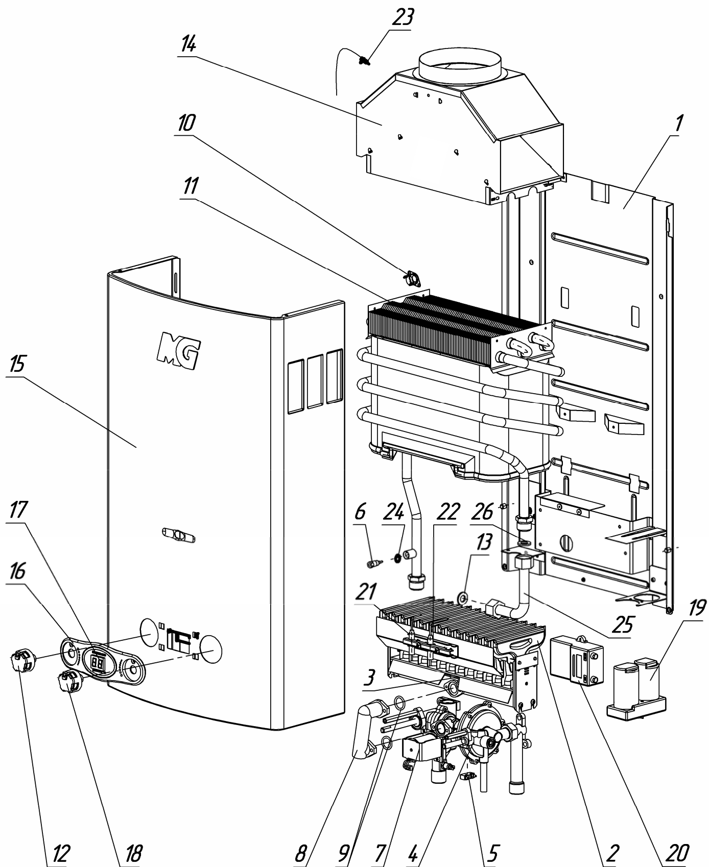
Рисунок 12. Вид аппарата с разнесенными частями
