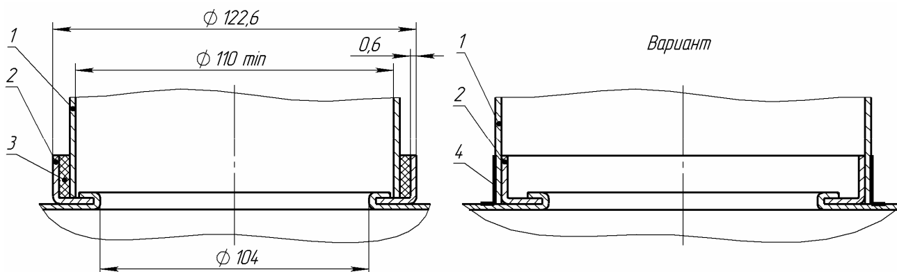
1 – газоотводящая труба; 2 – патрубок газоотводящего устройства; 3 – уплотнитель термостойкий; 4 – скотч алюминиевый термостойкий.
